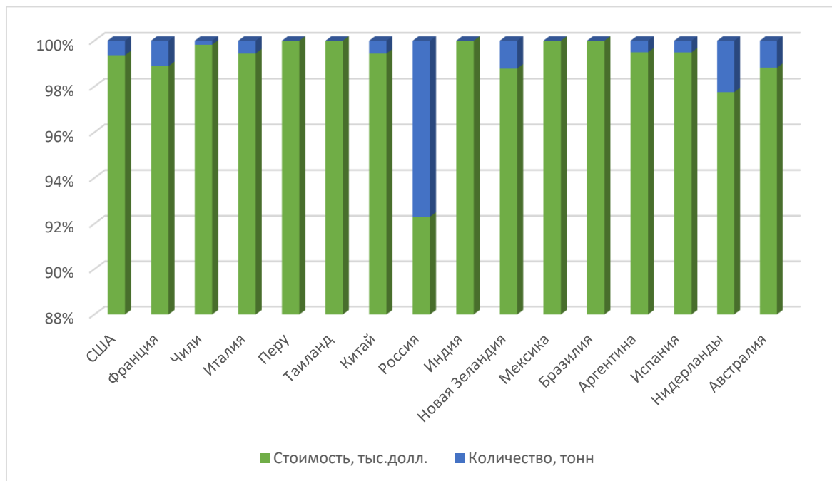
Диаграмма 46. Соотношение стоимости и количества, импортируемого 120991 – Семена овощей, 2018 г.
