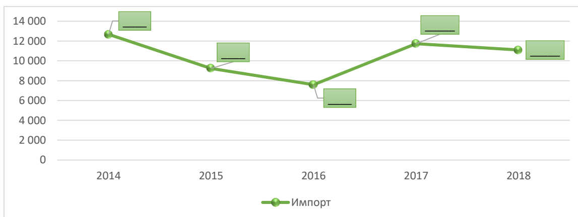
Диаграмма 45. Динамика импорта 120991 – Семена овощей, тыс.долл
